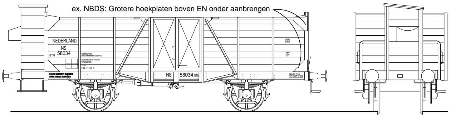
1921-1955: Set T-50p2 (alleen grijze wagens mogelijk) Afgebeeld: NBDS wagon na ombouw in 1925 met ouder model remhuis. Ook zonder spaakwielen mogelijk
