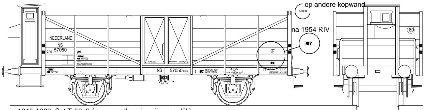
1945-1960: Set T-50p3 (wagens alleen in grijs mogelijk) Afgebeeld: Standaard uitvoering vanaf 1945 Varianten: ander model wagon, al dan niet met remhuis
