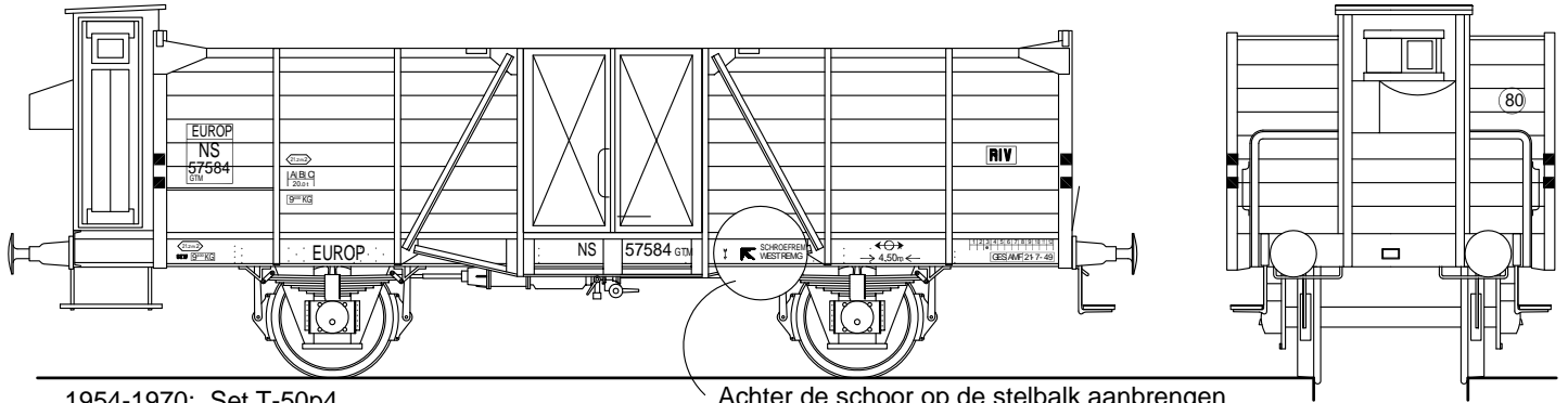
1954-1970: Set T-50p4 Afgebeeld: Europ wagon, in grijs (tot 1970) en roodbruin mogelijk. Varianten: ander model wagon, al dan niet met remhuis. Ook zonder Europ kader mogelijk (alleen NS en nummer eronder)
