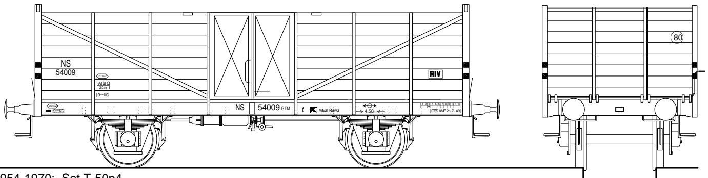
1954-1970: Set T-50p4 Afgebeeld: Standaard uitvoering, in grijs (tot 1970) en roodbruin mogelijk. Varianten: ander model wagon, al dan niet met remhuis
